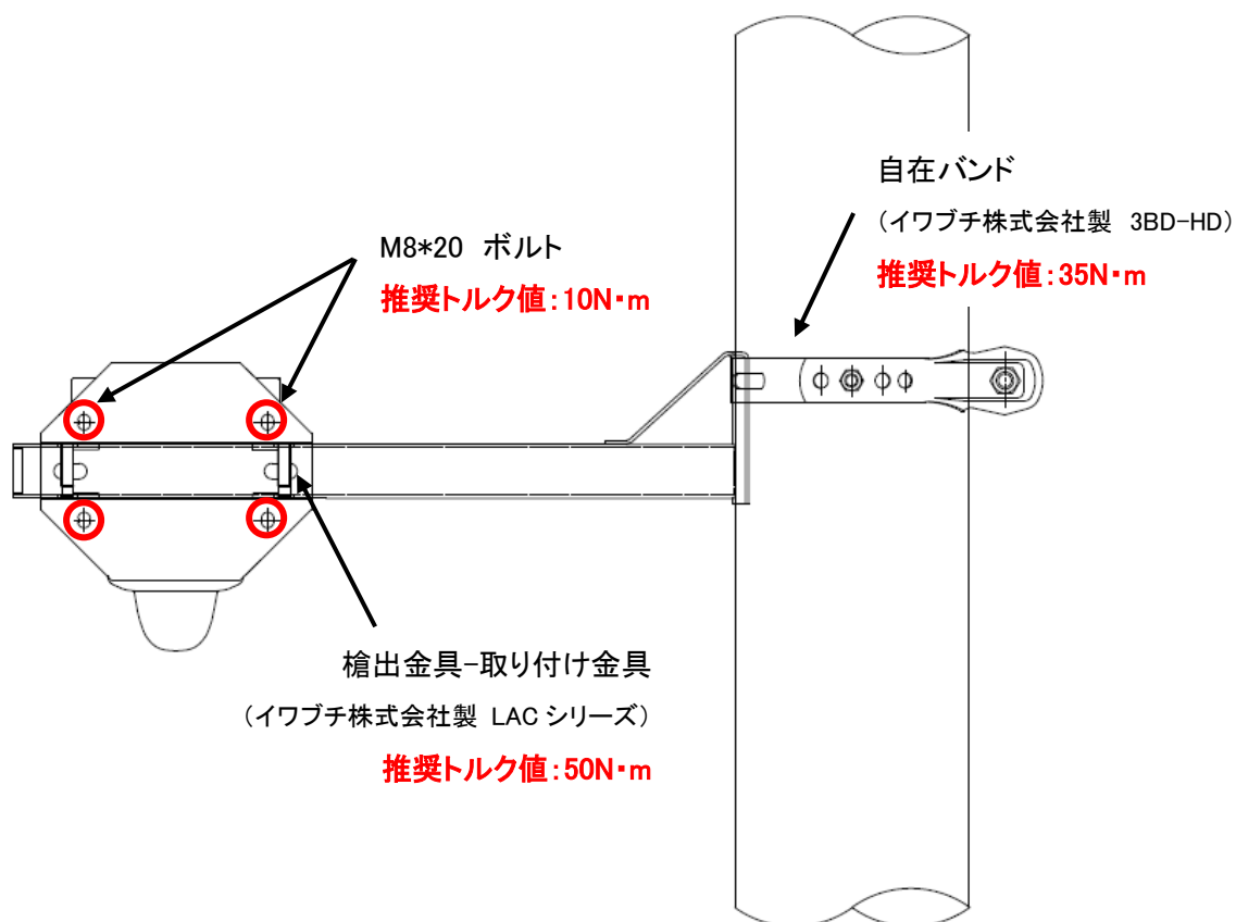
<< 設置図 側面 >>
