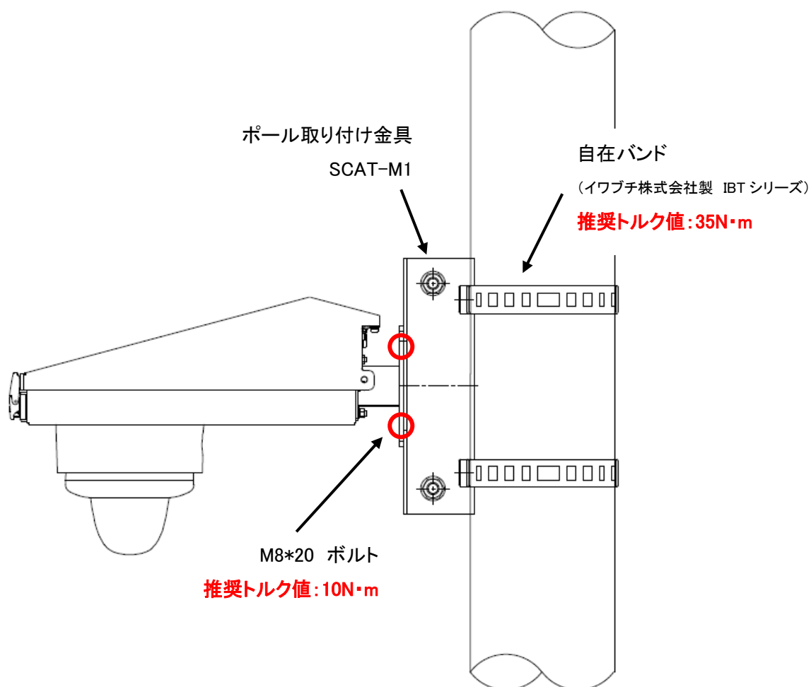
<< 設置図 側面 >>
