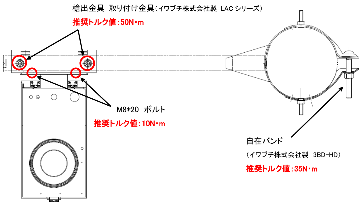
<< 設置図 下面 >>
