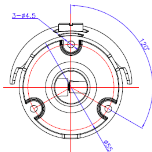
取付面
