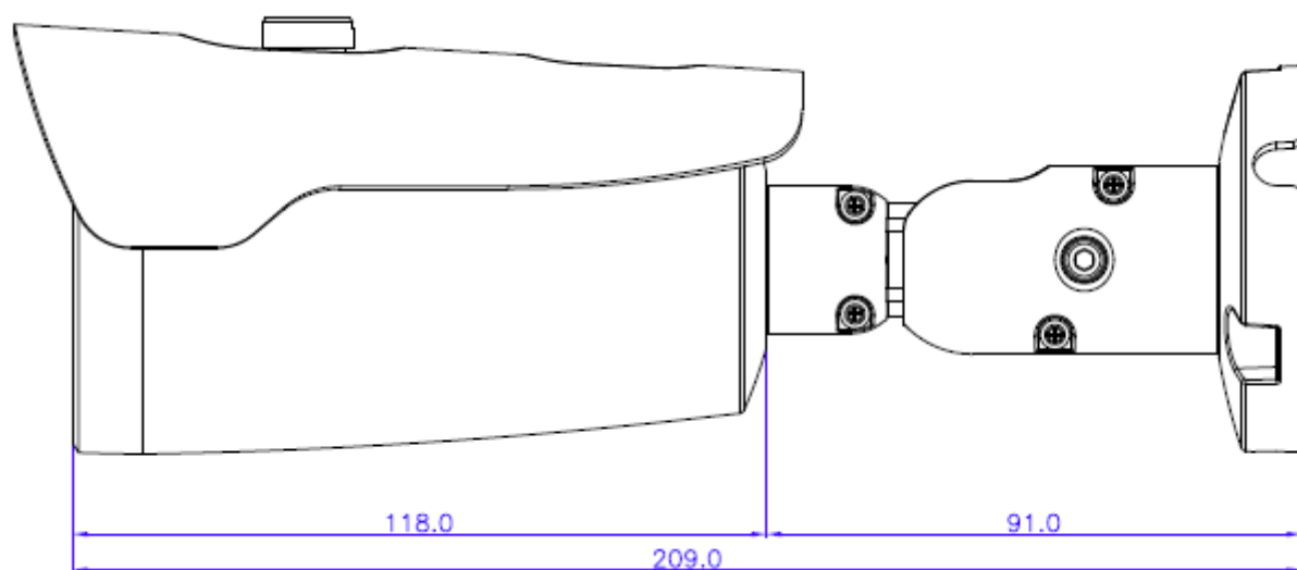
側面
