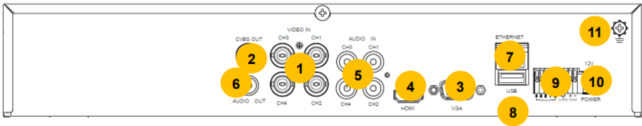
背面パネルの各ボタン説明
