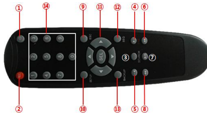
リモコンの各ボタン説明
